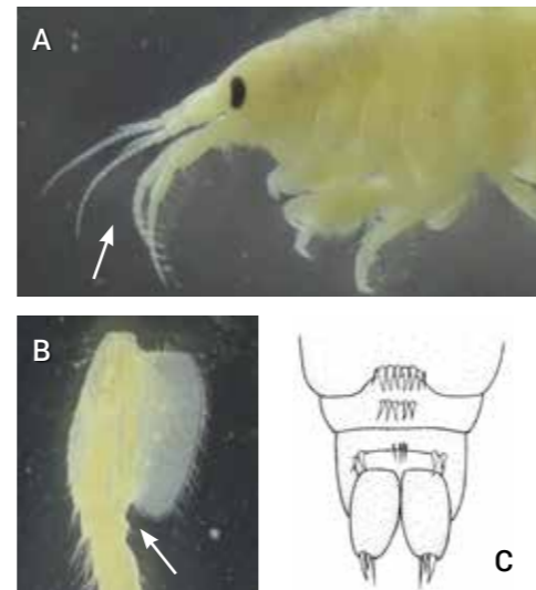
3. attēls. Līdzīgās sugas Pontogammarus robustoides (A) antenas, (B) 5. krūšņķas augšējā locītava un (C) vēdera urosomālie segmenti.
