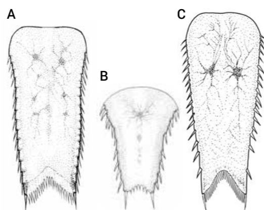
2. attēls. Līdzīgo sugu Paramysis lacustris (A), Limnomysis benedeni (B) un Mysis relicta (C) telsoni ILUSTR. ALEKSANDRS ANIŠČENKO
