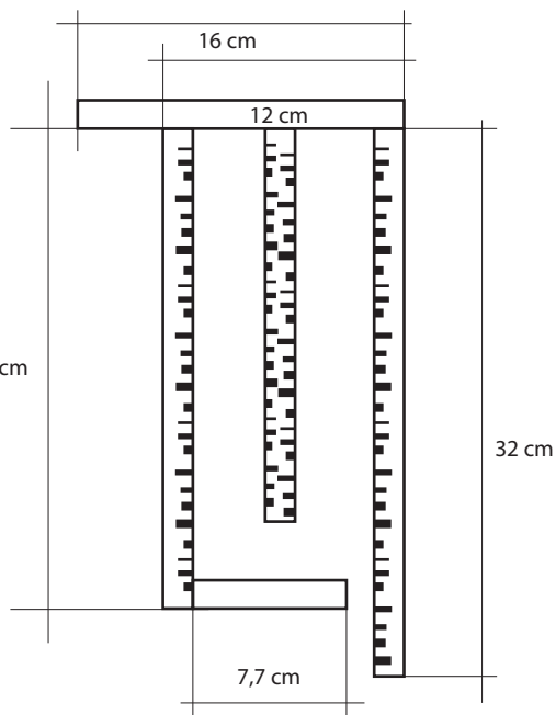
SĀNSKATS /šķērsgriezums/
